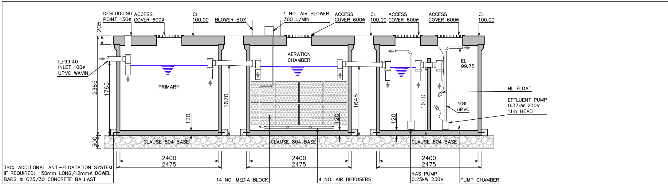
SECTION A-A
