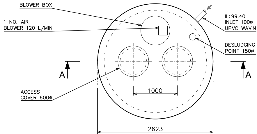
LID PLAN
