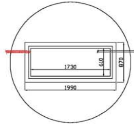
Lid Plan
